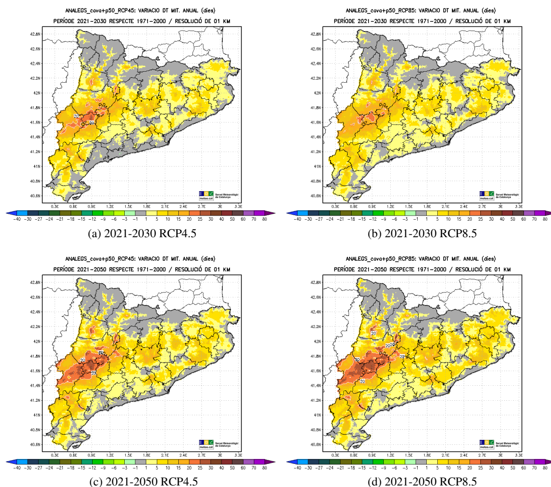
Figura 5.84: Variació projectada (en dies) del nombre mitjà anual de Dies Tòrrids (DT, dies amb TX \geq 35^\circ C ) respecte al període de referència 1971-2000, per als períodes 2021-2030 (dalt) i 2021-2050 (baix) i els escenaris d'emissions RCP4.5 (esquerra) i RCP8.5 (dreta).
