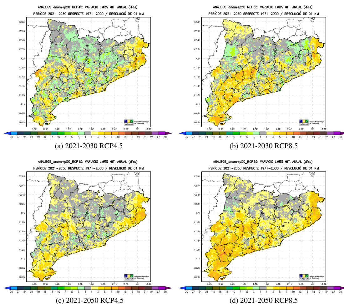
Figura 5.92: Variació projectada (en dies) de la Longitud Màxima de la Ratxa Seca (LMRS, nombre màxim de dies consecutius amb PPT < 1 mm) anual respecte al període de referència 1971-2000, per als períodes 2021-2030 (dalt) i 2021-2050 (baix) i els escenaris d'emissions RCP4.5 (esquerra) i RCP8.5 (dreta).
