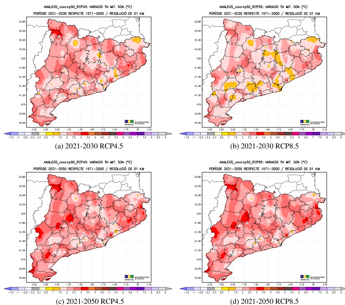
Figura 5.72: Variació projectada (en °C) de la Temperatura Mínima (TN) mitjana de tardor (SON) respecte al període de referència 1971-2000, per als períodes 2021-2030 (dalt) i 2021-2050 (baix) i els escenaris d'emissions RCP4.5 (esquerra) i RCP8.5 (dreta).
