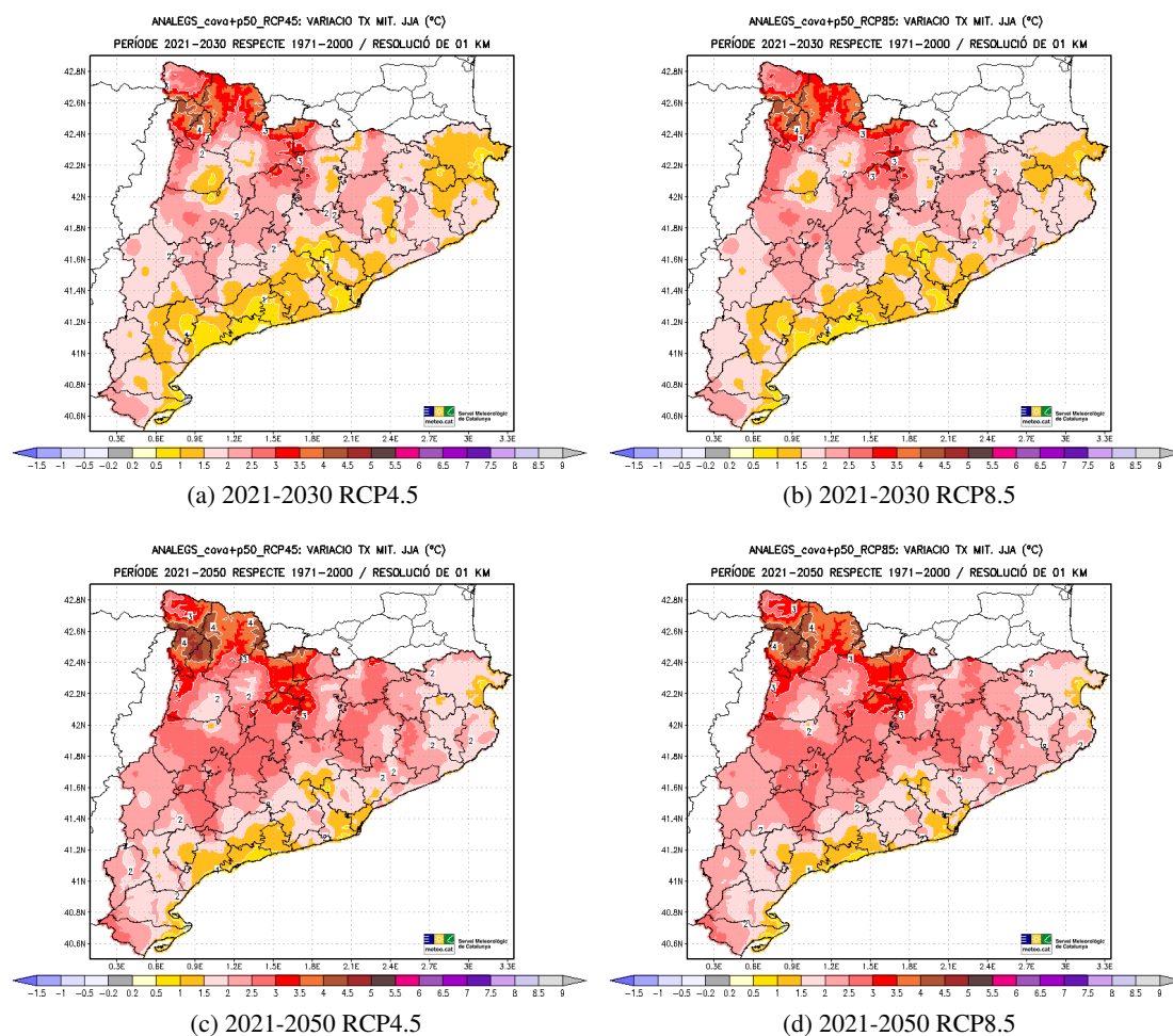
Figura 5.76: Variació projectada (en °C) de la Temperatura Màxima (TX) mitjana d'estiu (JJA) respecte al període de referència 1971-2000, per als períodes 2021-2030 (dalt) i 2021-2050 (baix) i els escenaris d'emissions RCP4.5 (esquerra) i RCP8.5 (dreta).
