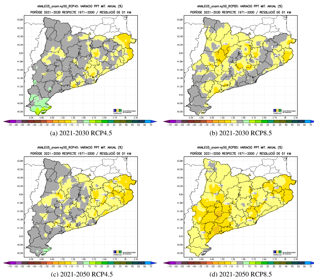
Figura 5.78: Variació projectada (en %) de la Precipitació (PPT) mitjana anual respecte al període de referència 1971-2000, per als períodes 2021-2030 (dalt) i 2021-2050 (baix) i els escenaris d'emissions RCP4.5 (esquerra) i RCP8.5 (dreta).
