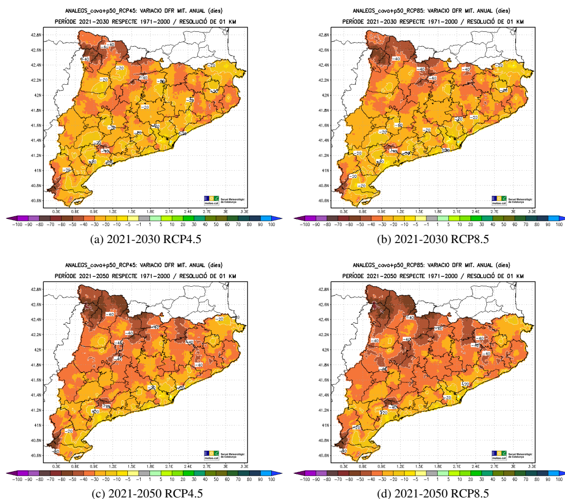
Figura 5.86: Variació projectada (en dies) del nombre mitjà anual de Dies de Fredor (DFR, dies amb TM \leq 10^{\circ}C ) respecte al període de referència 1971-2000, per als períodes 2021-2030 (dalt) i 2021-2050 (baix) i els escenaris d'emissions RCP4.5 (esquerra) i RCP8.5 (dreta).
