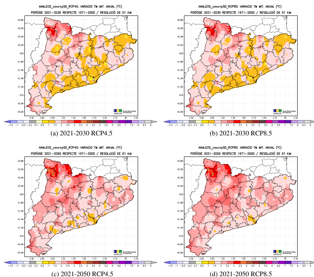
Figura 5.63: Variació projectada (en °C) de la Temperatura Mitjana (TM) anual respecte al període de referència 1971-2000, per als períodes 2021-2030 (dalt) i 2021-2050 (baix) i els escenaris d'emissions RCP4.5 (esquerra) i RCP8.5 (dreta).
