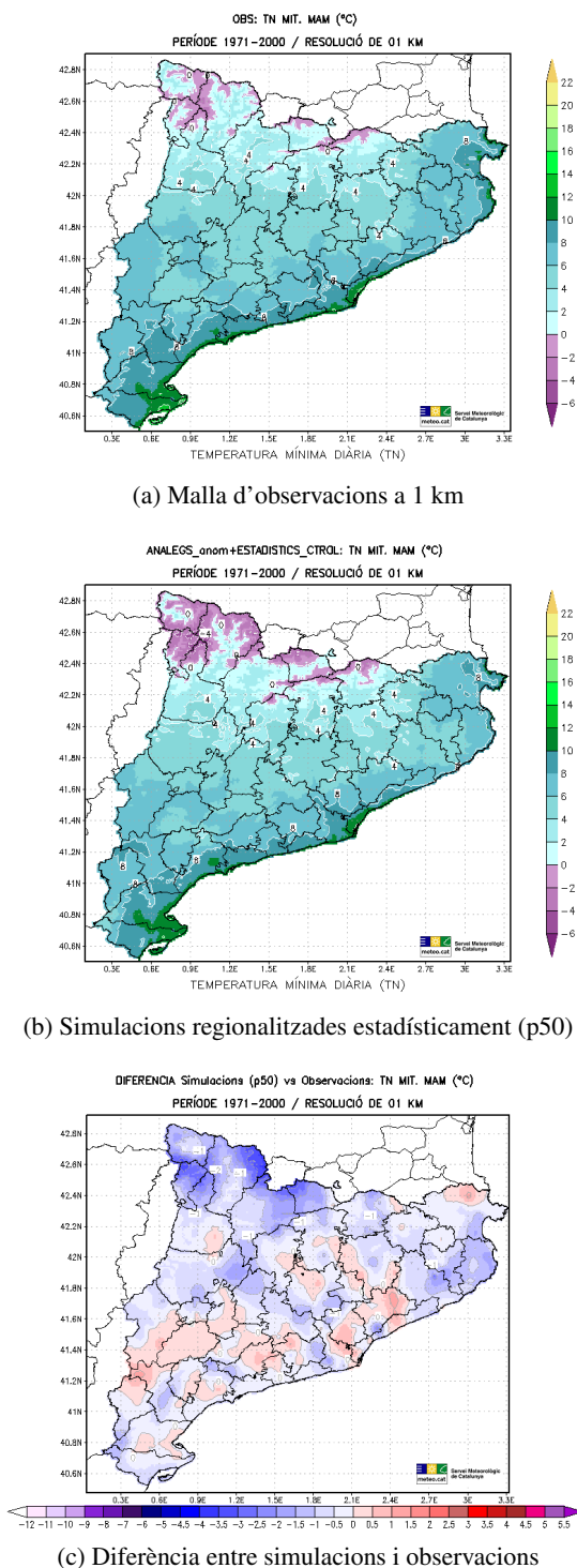
Figura 5.8: Camps espacials (en °C) de la temperatura mínima (TN) mitjana de primavera (MAM) per al període de control (1971-2000) a Catalunya segons: a) la malla d'observacions a 1 km, b) el percentil 50 (p50) de les simulacions regionalitzades estadísticament i c) la diferència entre els dos camps anteriors (valors simulats menys observats).
