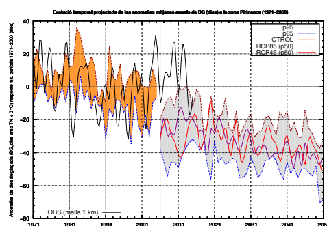
Figura 5.54: Evolució temporal projectada (1971-2100) de les anomalies mitjanes anuals (en dies) del nombre total de dies de glaçada (DG, dies amb TN \leq 0^\circ C ) respecte el valor mitjà del període de control (1971-2000) per al conjunt de Catalunya (a), zona litoral i prelitoral (b), zona interior (c) i zona pirinenca (d).
