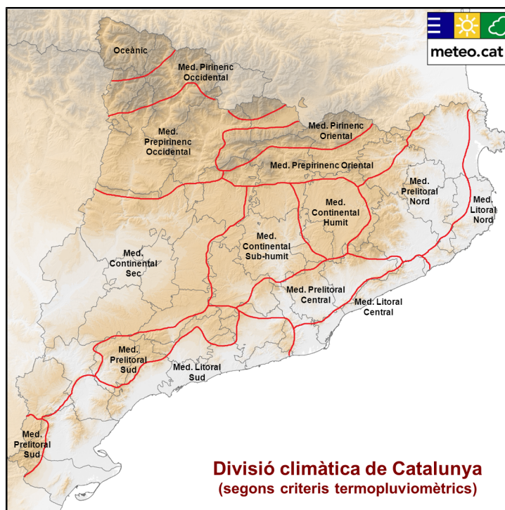
Figura 2.2: Divisió climàtica de Catalunya seguint criteris termopluviomètrics.
