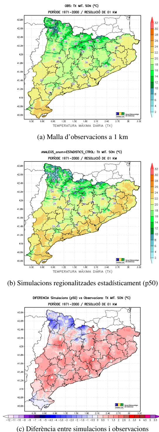
Figura 5.15: Camps espacials (en °C) de la temperatura màxima (TX) mitjana de tardor (SON) per al període de control (1971-2000) a Catalunya segons: a) la malla d'observacions a 1 km, b) el percentil 50 (p50) de les simulacions regionalitzades estadísticament i c) la diferència entre els dos camps anteriors (valors simulats menys observats).
