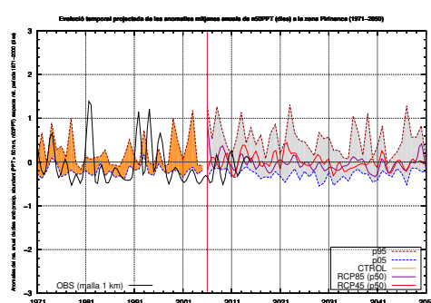
Figura 5.60: Evolució temporal projectada (1971-2050) de les anomalies mitjanes anuals (en dies) del nombre total de dies amb precipitació abundant (n50PPT, dies amb PPT \geq 50 mm) respecte el valor mitjà del període de control (1971-2000) per al conjunt de Catalunya (a), zona litoral i prelitoral (b), zona interior (c) i zona pirinenca (d).
