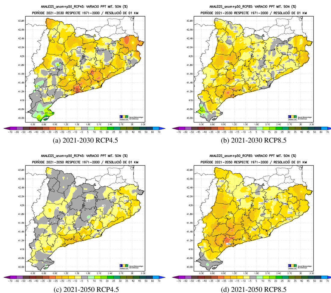
Figura 5.82: Variació projectada (en %) de la Precipitació (PPT) mitjana de tardor (SON) respecte al període de referència 1971-2000, per als períodes 2021-2030 (dalt) i 2021-2050 (baix) i els escenaris d'emissions RCP4.5 (esquerra) i RCP8.5 (dreta).
