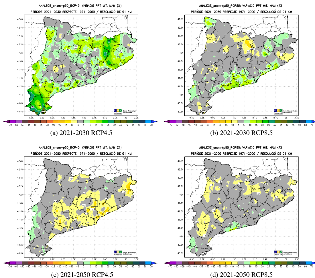
Figura 5.80: Variació projectada (en %) de la Precipitació (PPT) mitjana de primavera (MAM) respecte al període de referència 1971-2000, per als períodes 2021-2030 (dalt) i 2021-2050 (baix) i els escenaris d'emissions RCP4.5 (esquerra) i RCP8.5 (dreta).
