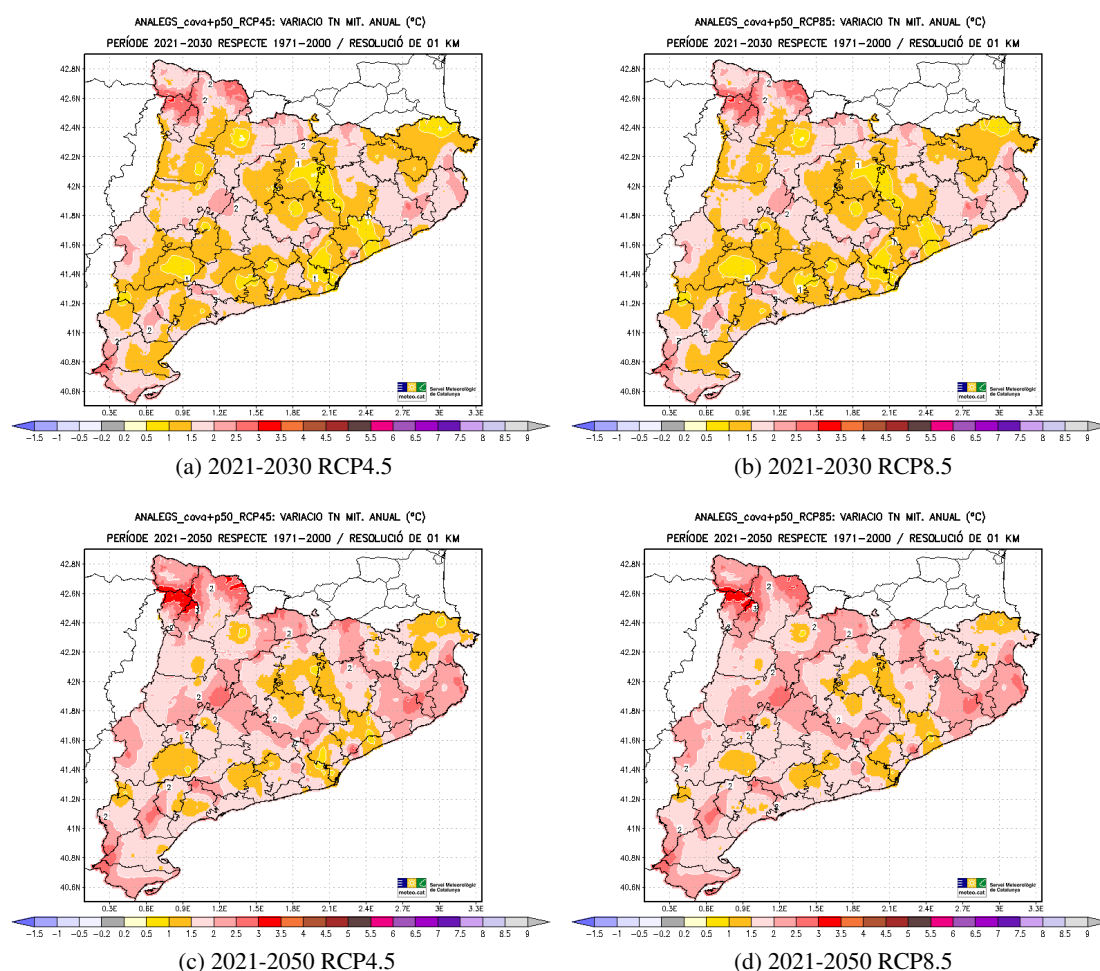
Figura 5.68: Variació projectada (en °C) de la Temperatura Mínima (TN) mitjana anual respecte al període de referència 1971-2000, per als períodes 2021-2030 (dalt) i 2021-2050 (baix) i els escenaris d'emissions RCP4.5 (esquerra) i RCP8.5 (dreta).
