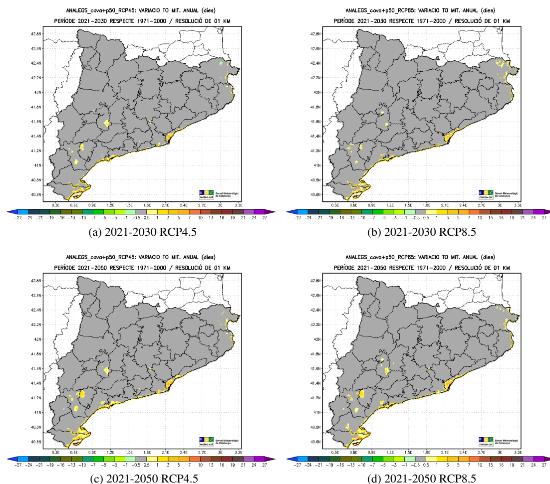
Figura 5.89: Variació projectada (en dies) del nombre mitjà anual de Nits Tòrrides (TO, dies amb TN \geq 25^{\circ}\text{C} ) respecte al període de referència 1971-2000, per als períodes 2021-2030 (dalt) i 2021-2050 (baix) i els escenaris d'emissions RCP4.5 (esquerra) i RCP8.5 (dreta).
