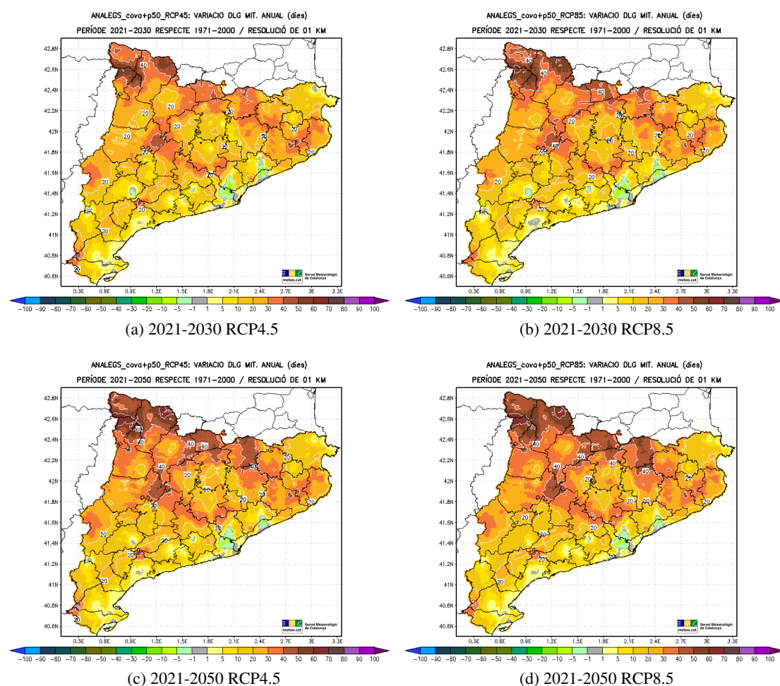
Figura 5.87: Variació projectada (en dies) del nombre mitjà anual de Dies Lliures de Glaçada (DLG, dies amb TN \geq 2^{\circ}C ) respecte al període de referència 1971-2000, per als períodes 2021-2030 (dalt) i 2021-2050 (baix) i els escenaris d'emissions RCP4.5 (esquerra) i RCP8.5 (dreta).
