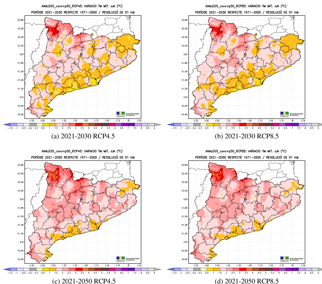
Figura 5.66: Variació projectada (en °C) de la Temperatura Mitjana (TM) d'estiu (JJA) respecte al període de referència 1971-2000, per als períodes 2021-2030 (dalt) i 2021-2050 (baix) i els escenaris d'emissions RCP4.5 (esquerra) i RCP8.5 (dreta).
