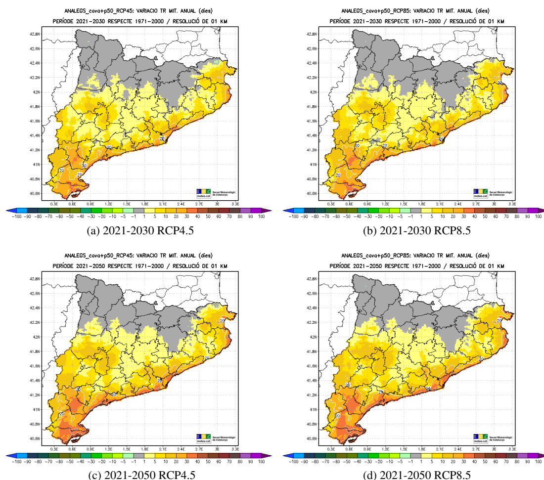
Figura 5.88: Variació projectada (en dies) del nombre mitjà anual de Nits Tropicals (TR, dies amb TN \geq 20^{\circ}C ) respecte al període de referència 1971-2000, per als períodes 2021-2030 (dalt) i 2021-2050 (baix) i els escenaris d'emissions RCP4.5 (esquerra) i RCP8.5 (dreta).
